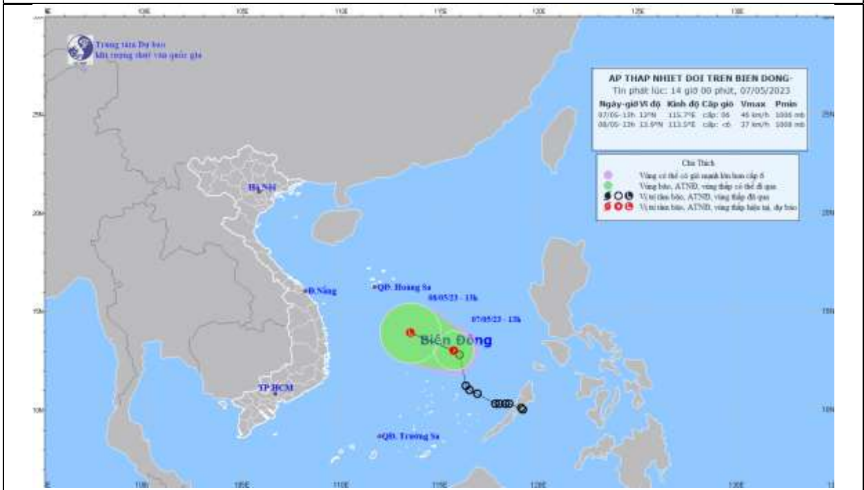
Hình 1. Bản đồ dự báo quỹ đạo và cường độ áp thấp nhiệt đới trên Biển Đông phát lúc 14h00 ngày 07/5/2023
